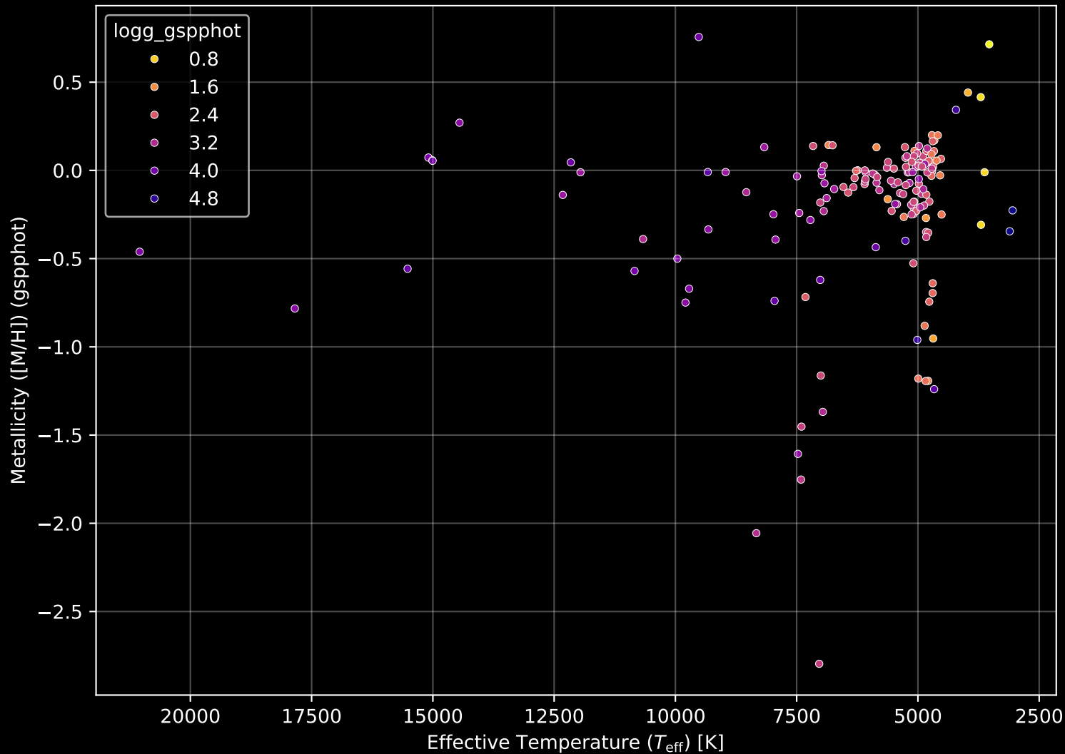
APOGEE DR17 Field: [105+00] Stellar Population Parameters (n= 157)
